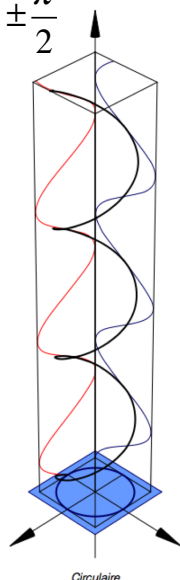
Doc. 10. Polarisations circulaires ( E_{0x} = E_{0y} = E_0 ).
