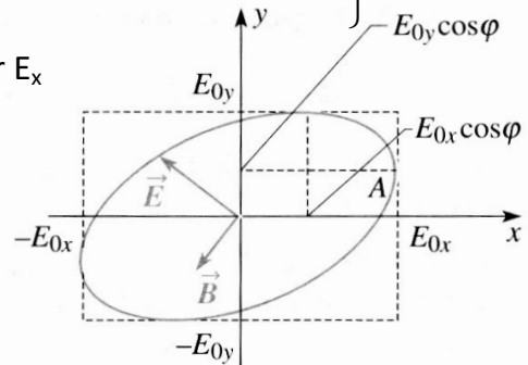
Polarisation elliptique. \left( \text{Cas } -\frac{\pi}{2} < \varphi < \frac{\pi}{2} \right)
