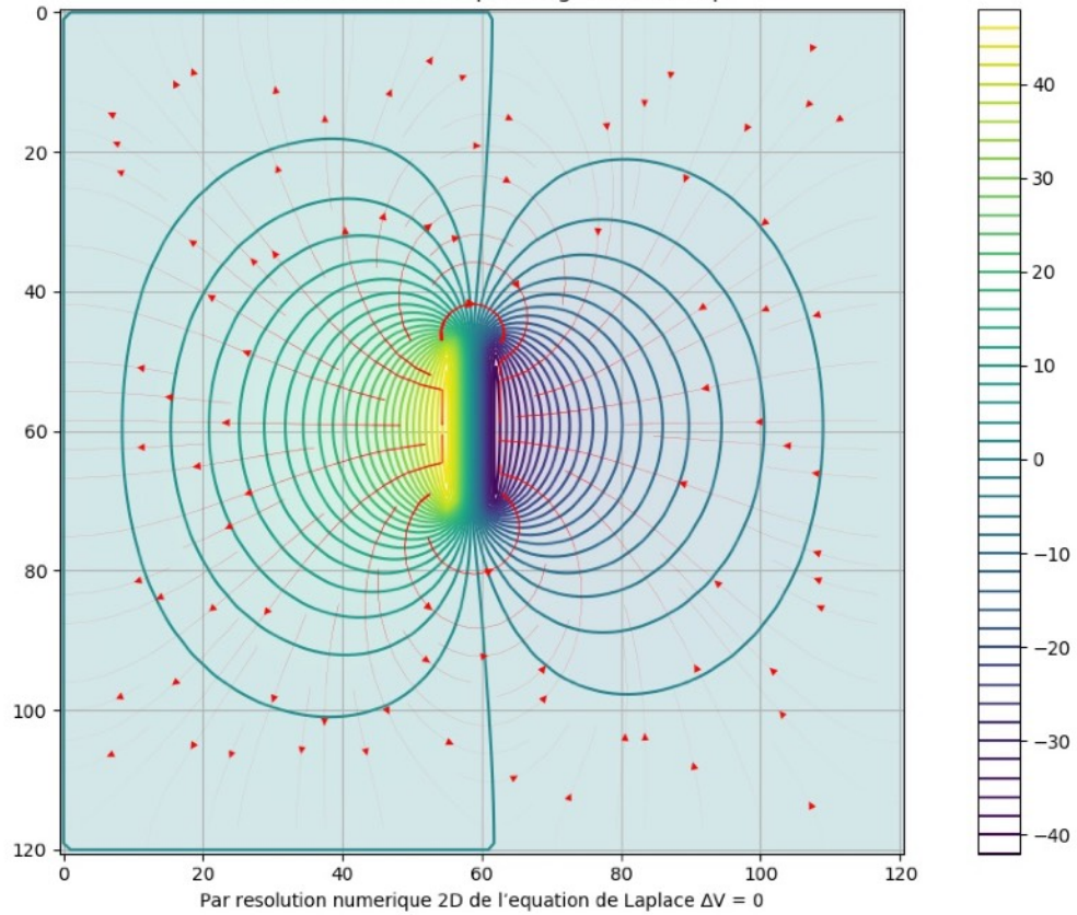
Potentiel electrostatique et lignes de champ
