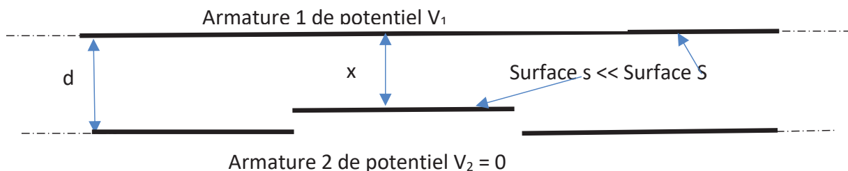
Figure 18 : modèle plan
