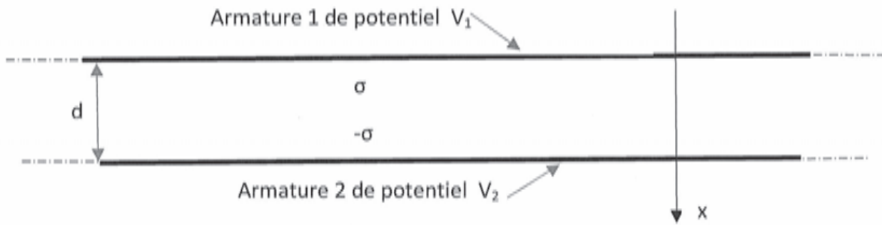
Figure 17 : condensateur plan
