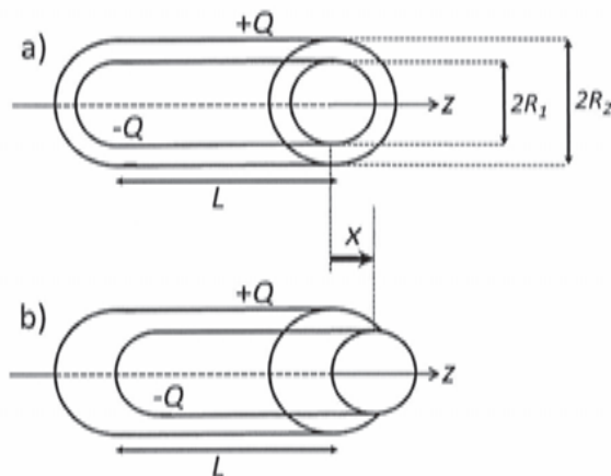
Fig. 2 : Condensateur cylindrique :
