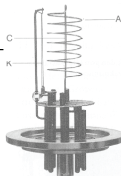
Figure B.4 : Sonde de Bayard-Alpert
